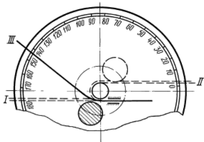
Схема испытания ленты на пружинность
