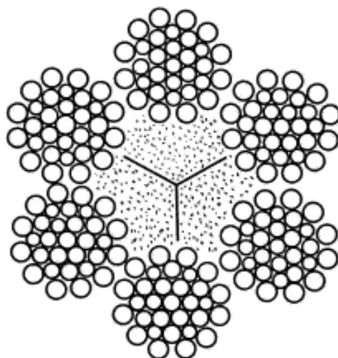
Шестипрядный канат 6×31+1 о. с.; 6×31=186 проволок с органическим сердечником (прядь каната 1+6+6/6+12).
