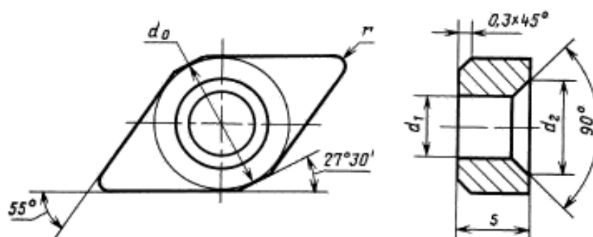
Размеры, мм
