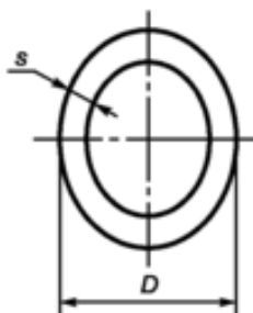
D — наружный диаметр; S — толщина стенки
